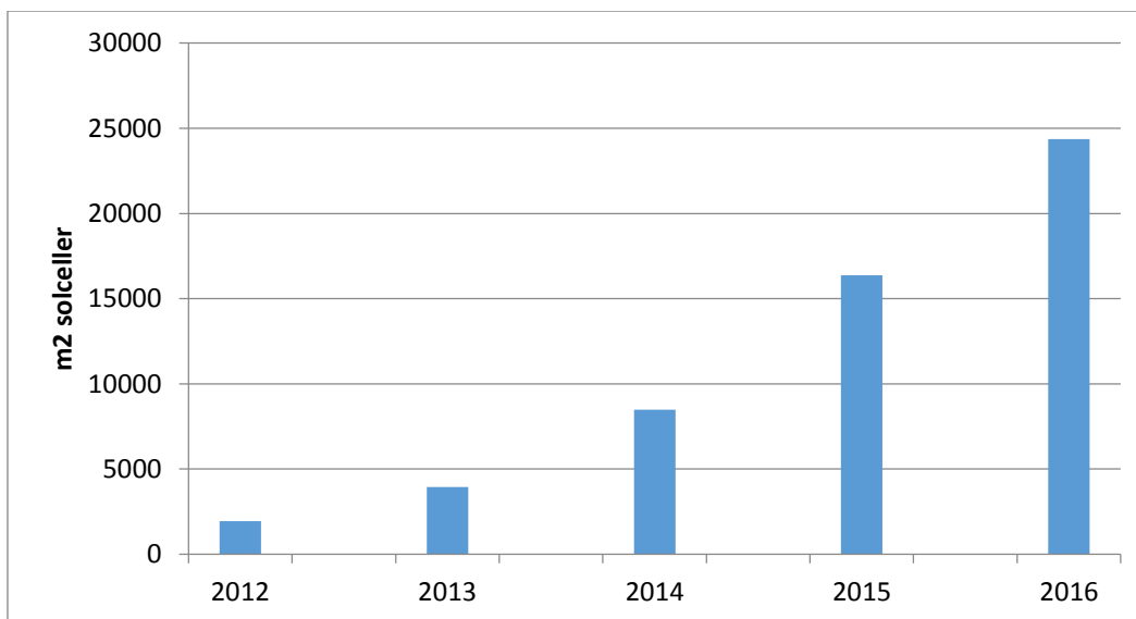
Figur 15. Solcellsutveckling i Jämtlands län
