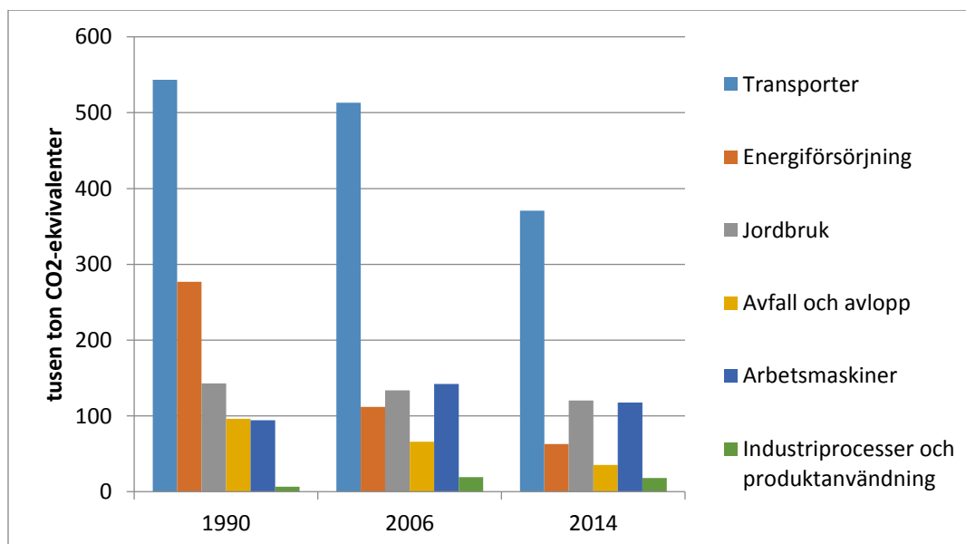
Figur 21. Utsläpp av växthusgaser per sektor i Jämtlands län under några år
